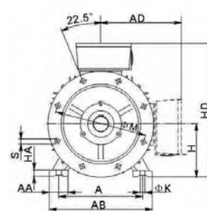
TAMAÑO 225-400
