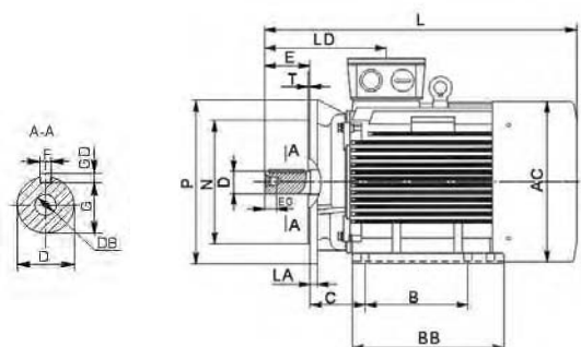
TAMAÑO 132-400
