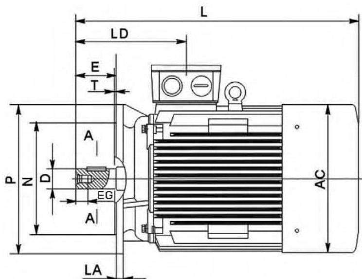
TAMAÑO 132-280
