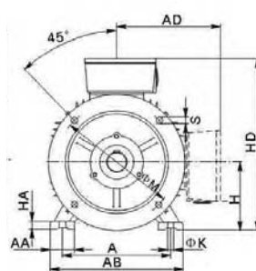
TAMAÑO 132-200
